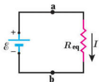
شکل ۲-۱۴ مدار معادل شکل ۲-۳۹ که در آن مقاومت معادل، R_{eq} جایگزین مقاومت‌های R_1, R_2, R_3 شده است.
