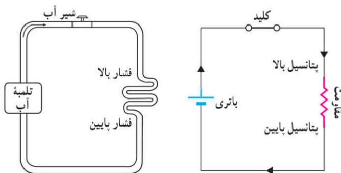
شکل ۲۸-۲ همان طور که تلمبه آب انرژی لازم برای شارش آب را فراهم می کند، باتری نیز انرژی لازم برای برقراری یک جریان را مهیا می سازد.
