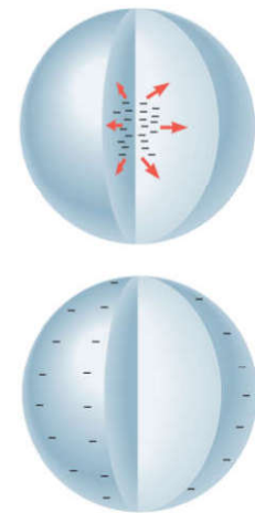
شکل ۱-۲۹ بار اضافی داده شده به یک رسانا در سطح خارجی آن توزیع می‌شود.
