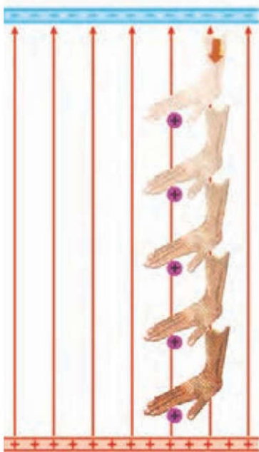
شکل ۳۷-۱ نیروی خارجی، بار +q را در خلاف جهت میدان الکتریکی جابه‌جا می‌کند.
