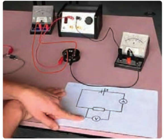
شکل ۸-۲ اسباب تحقیق قانون اهم. توجه کنید که آمپرسنج در مدار به صورت متوالی و ولت سنج به صورت موازی بسته شده است.
