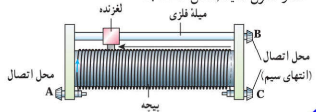
(الف) طرحی از ساختار یک رتوستای خطی
