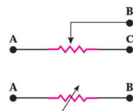
(ب) نماد یک رتوستا یا پتانسیومتر در مدار الکتریکی
