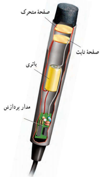
شکل ۱-۴۴ در یک میکروفون خازنی، با ارتعاش صفحه متحرک (دیفراگم) خازن بر اثر صدا، فاصله صفحه‌های خازن تغییر می‌کند بنابراین ظرفیت خازن تخت تغییر می‌کند که به ایجاد یک سیگنال الکتریکی می‌انجامد.
