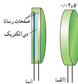
شکل ۱-۴۱ الف) بیرون و ب) درون یک خازن که بین صفحه‌های فلزی آن لایه عایقی قرار گرفته است.
