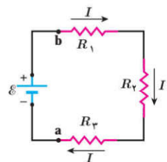
شکل ۲-۳۶ سه مقاومت که به طور متوالی به یک باتری آرمانی متصل شده‌اند.
