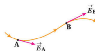
شکل ۱۵-۱ میدان الکتریکی در هر نقطه برداری است مماس بر خط میدانی که از آن نقطه می‌گذرد و با آن خط میدان هم جهت است.
