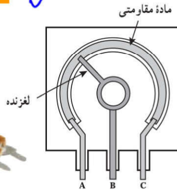
(ث) طرحی از یک پتانسیومتر
