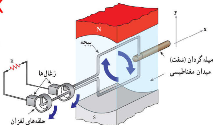
شکل ۴-۱۴ اجزای یک مولد (ژنراتور) جریان متناوب. حرکت مکانیکی از طریق میله گردان، سبب چرخیدن پیچه در میدان مغناطیسی می‌شود و جریان متناوبی را در مدار به وجود می‌آورد.
