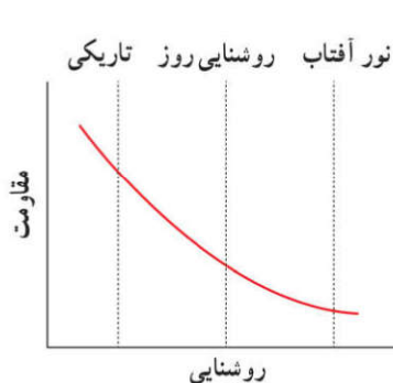
شکل ۲-۲ مقاومت بر حسب روشنایی برای یک LDR نوعی
