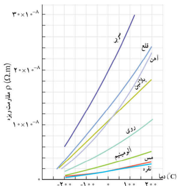
شکل ۱۴-۲ نمودار مقاومت ویژه چند فلز در یک گستره دمایی
