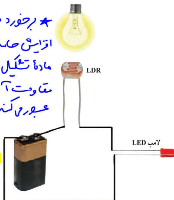
شکل ۲-۲ یک مدار ساده متشکل از یک LDR، یک باتری، و یک لامپ LED. با روشن شدن چراغ روشنایی لامپ LED روشن می‌شود.
